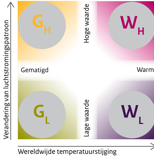
Figuur 1.11 KNMI'14-klimaatscenario's
